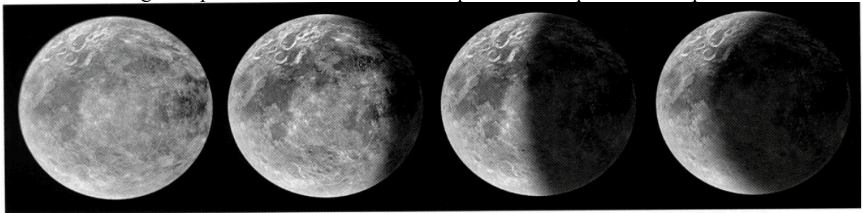
Document 2 : Les phases lunaires
