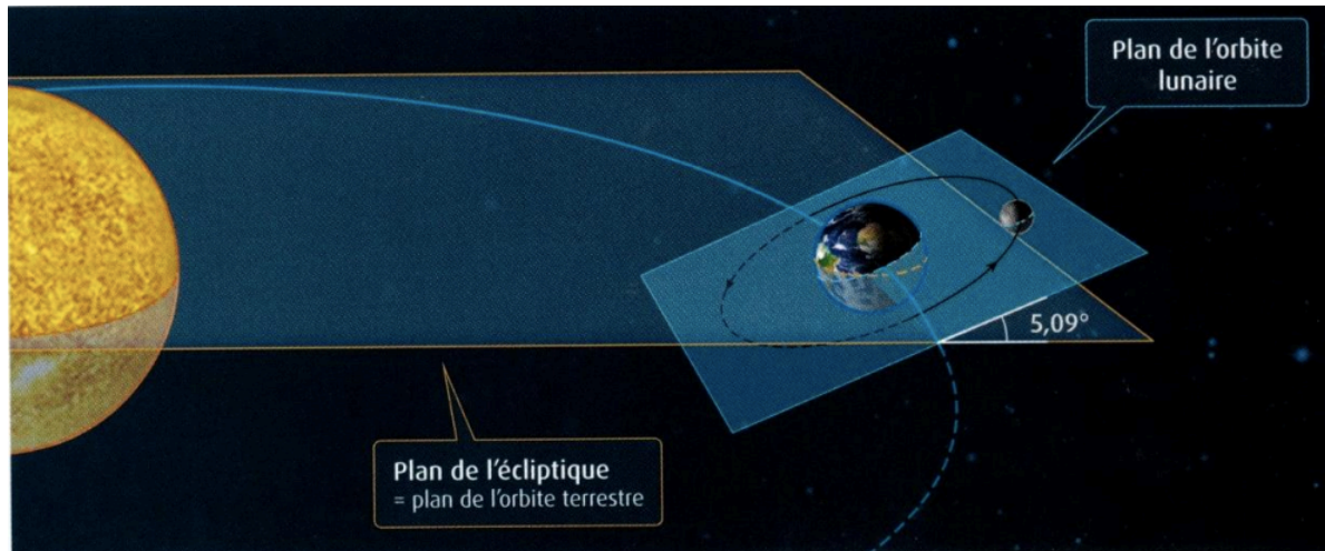
Document 1 : Plans des orbites terrestres et Lunaires
